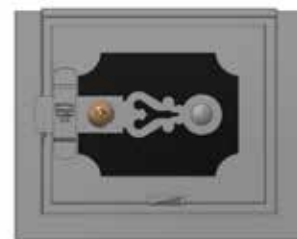
3003.00 Topné dvířko 31x25
