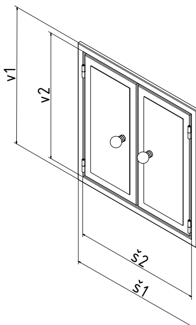
3410.03 Dvoukřídlé dvířko 42x46
